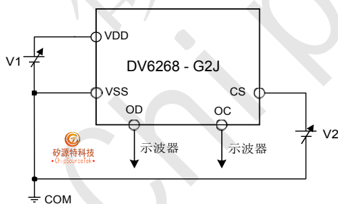
图 7: (测试电路 5)
