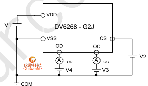
图 6: (测试电路 4)
