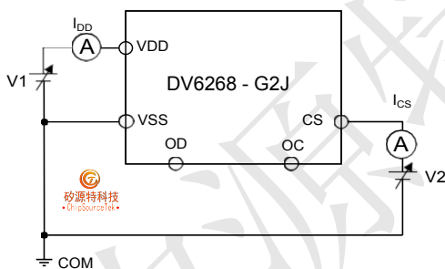
图 5: (测试电路 3)
