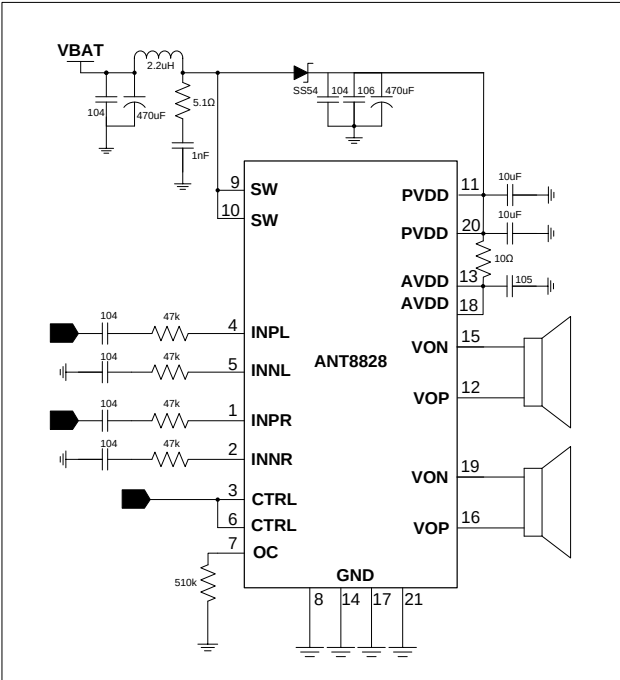
图 1 典型应用电路图
