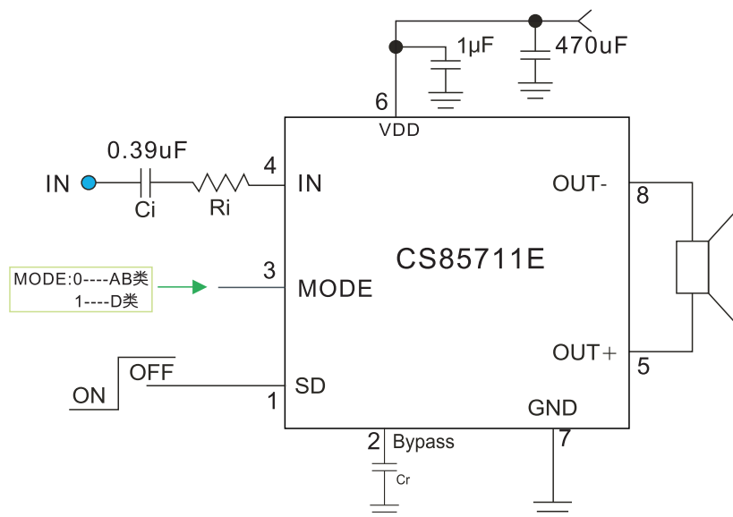
CS85711应用电路图
