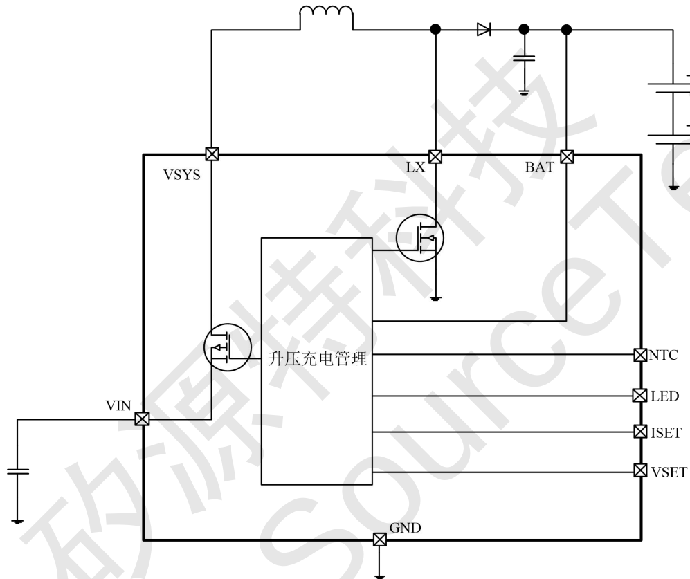
图 3 CST2342 内部框图
