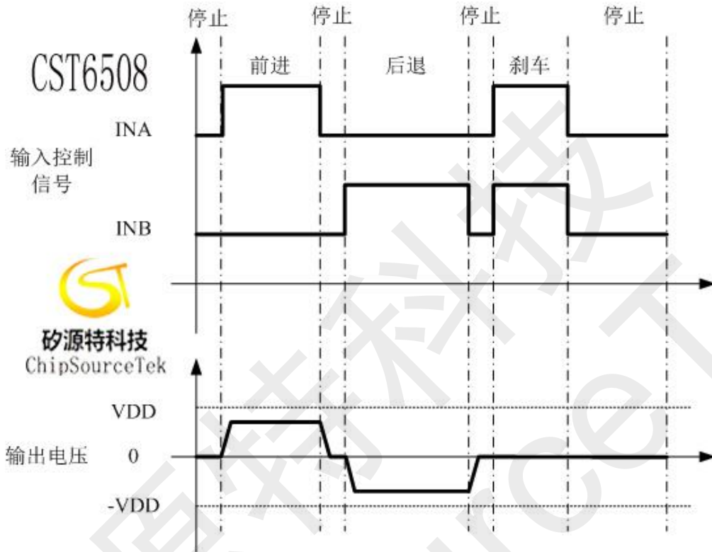
CST6508 工作波形图
