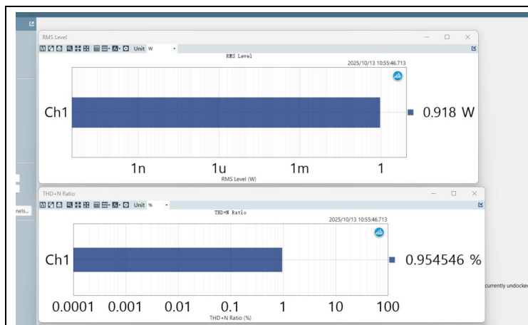
CST8302S 3.3V 4 欧 1%
