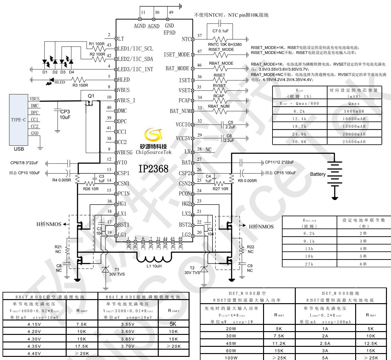
图 13 应用原理图
