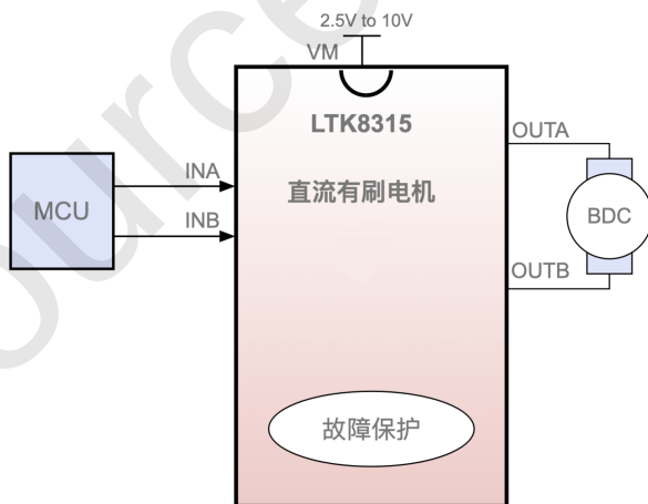
图1. LTK8315典型应用原理图
