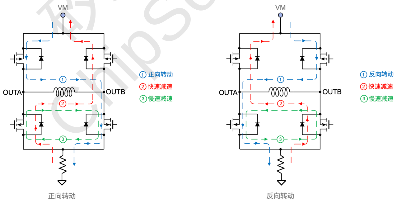
图4. 驱动和衰减模式
