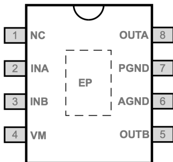
图2. LTK8315管脚说明
