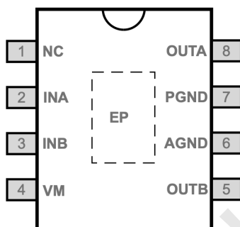
图2. LTK8530管脚说明
