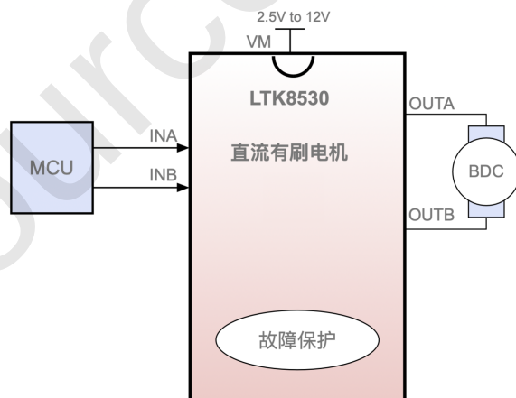
图1. LTK8530典型应用原理图
