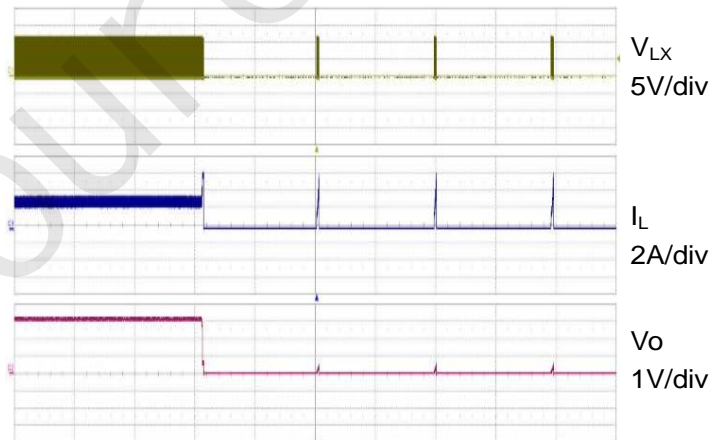
Fig.7 短路保护 20ms/div
