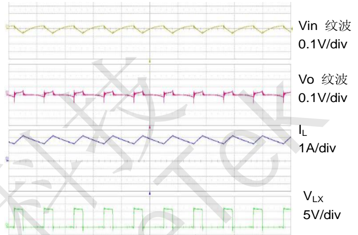
Fig.5 满载工作 2µs/div
