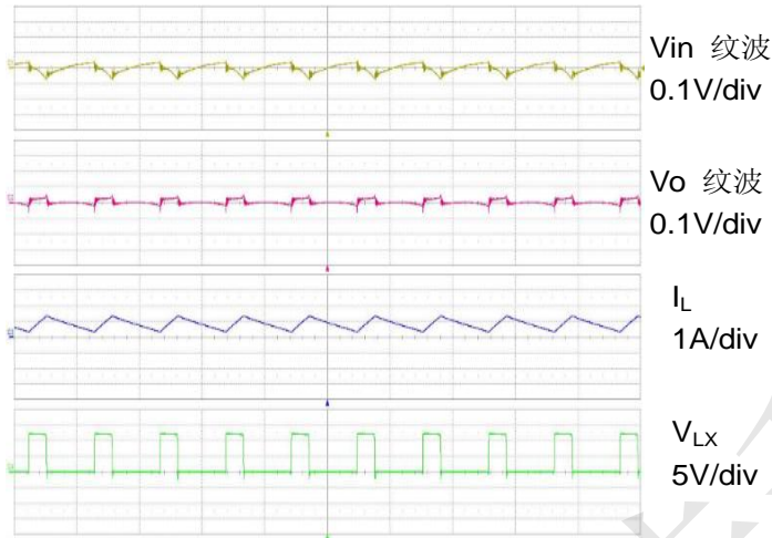
Fig.4 轻载工作 2µs/div
