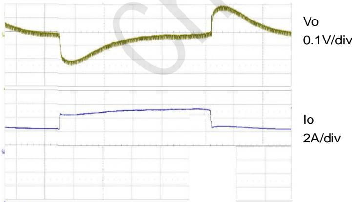
Fig.8 50% 到 100%负载瞬态 10µs/div
