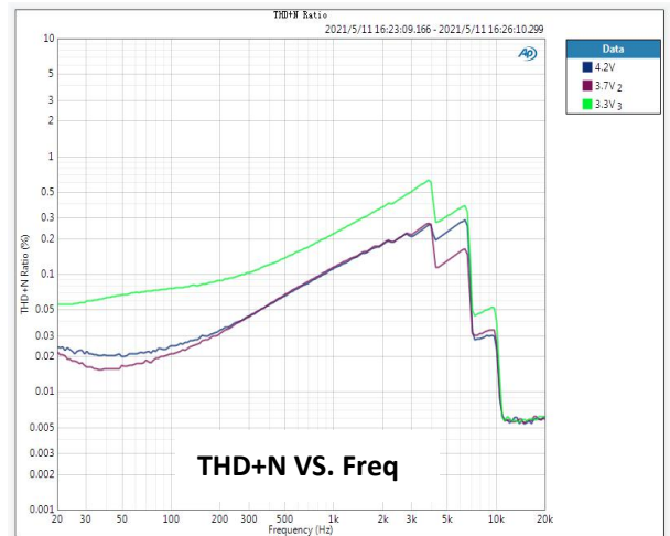
R_L=2\text{ohm} , Class AB
