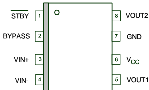
TS4990IDT - SO-8
