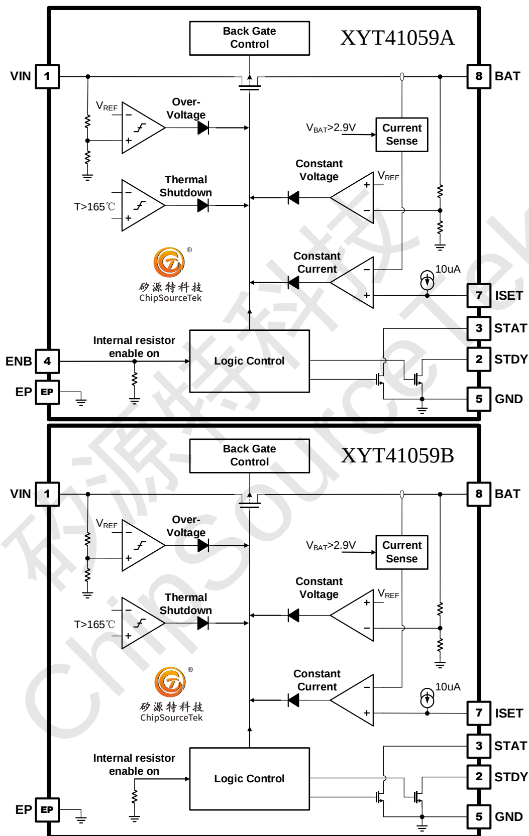
图 2 XYT41059模块功能框图
