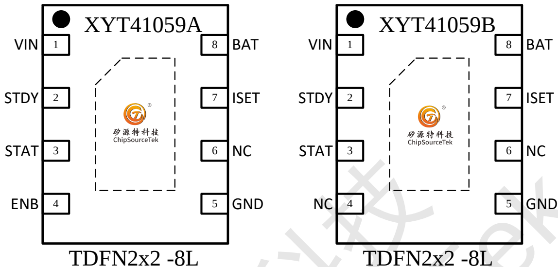
图1 XYT41059A/B管脚顶视图
