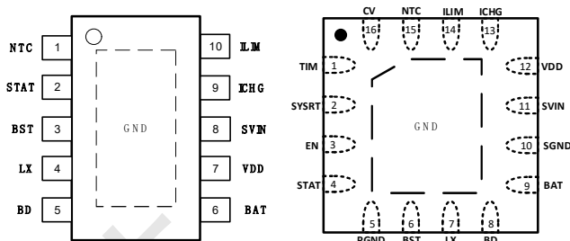
图3. 引脚排列
