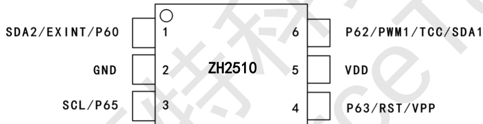
ZH2510-6PIN 脚位图
