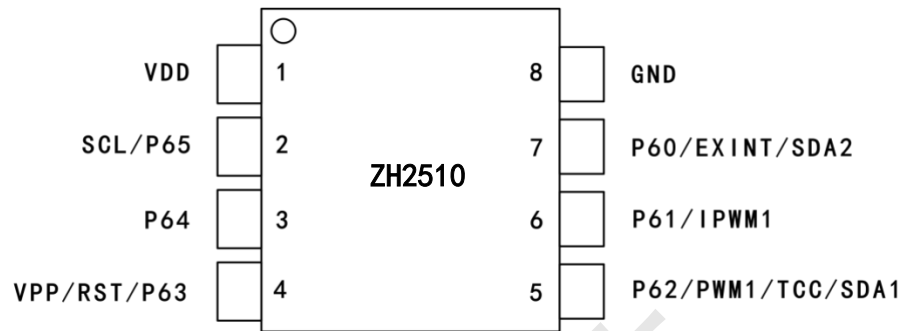
ZH2510-8PIN 脚位图
