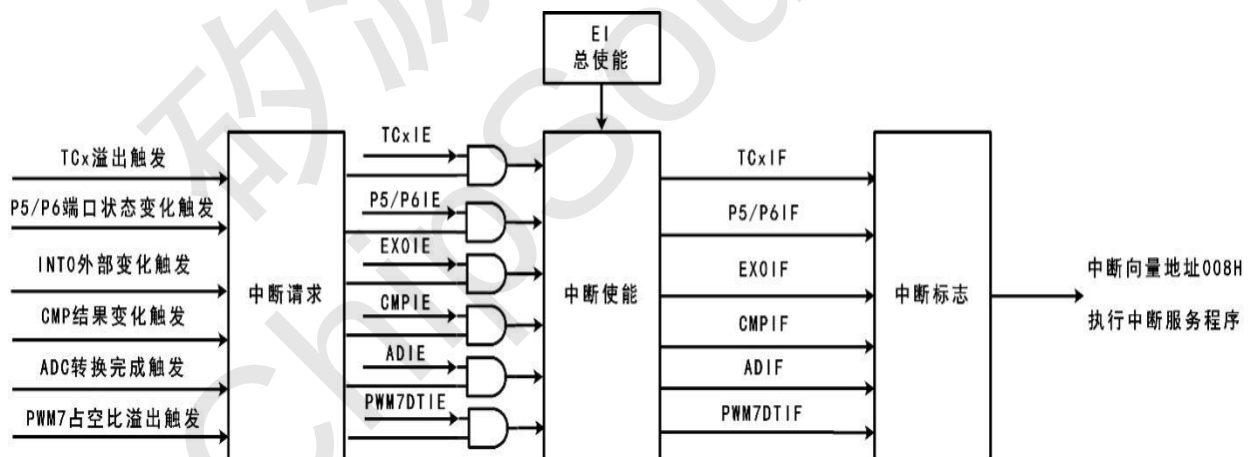
中断原理示意图
