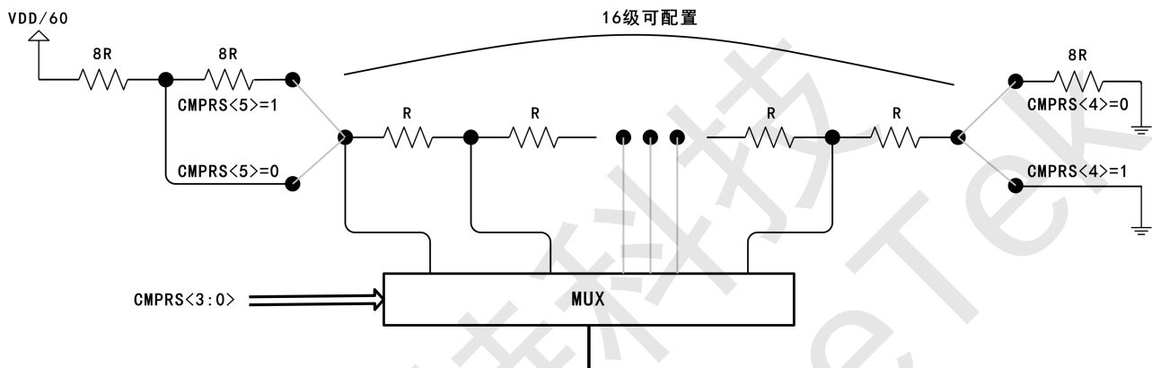
比较器修调示意图
