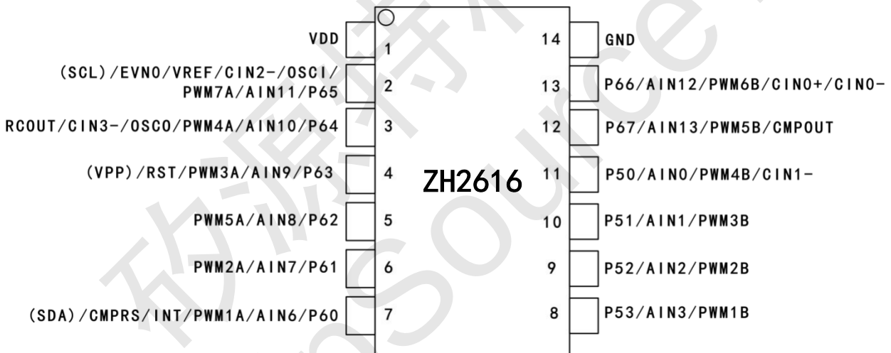
ZH2616-14PIN 脚位图
