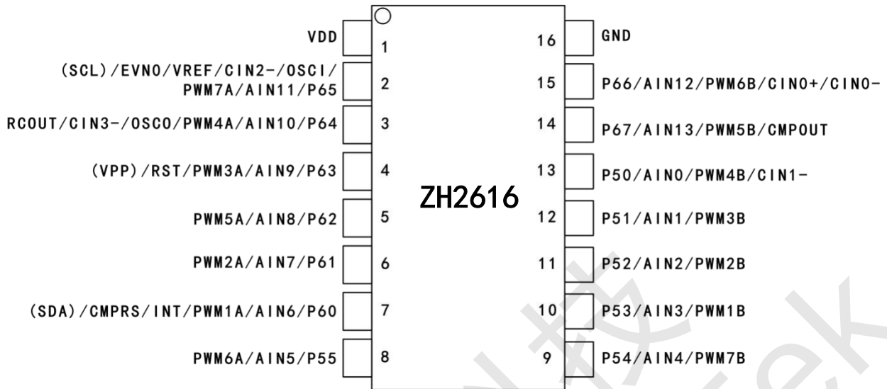
ZH2616-16PIN 脚位图
