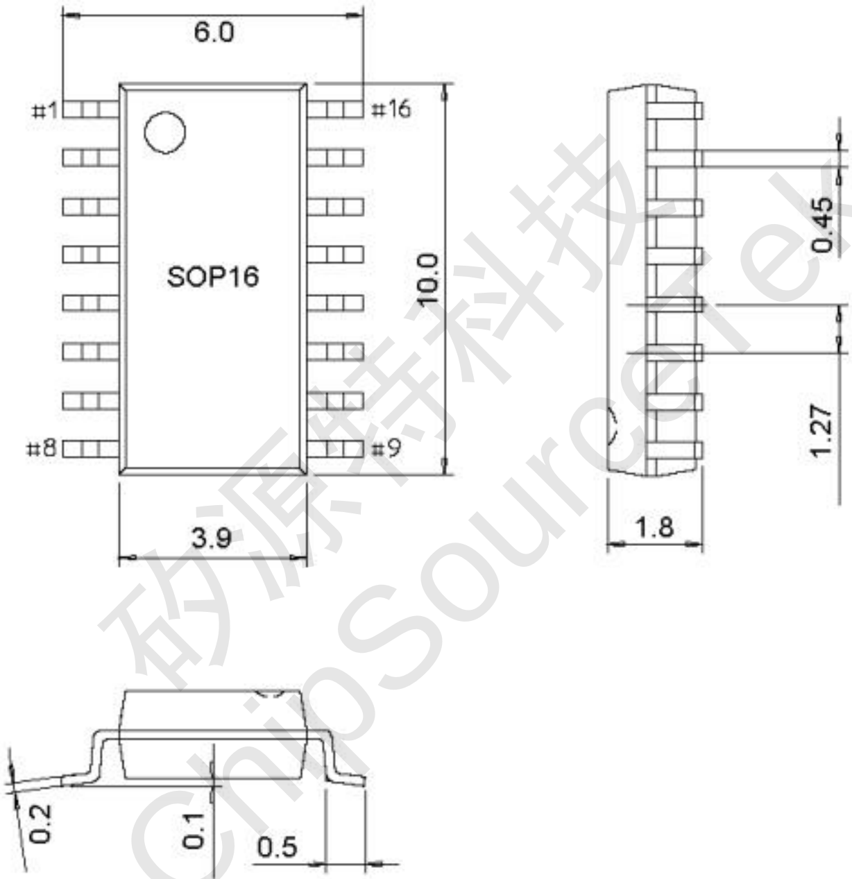
SOP16 封装尺寸
