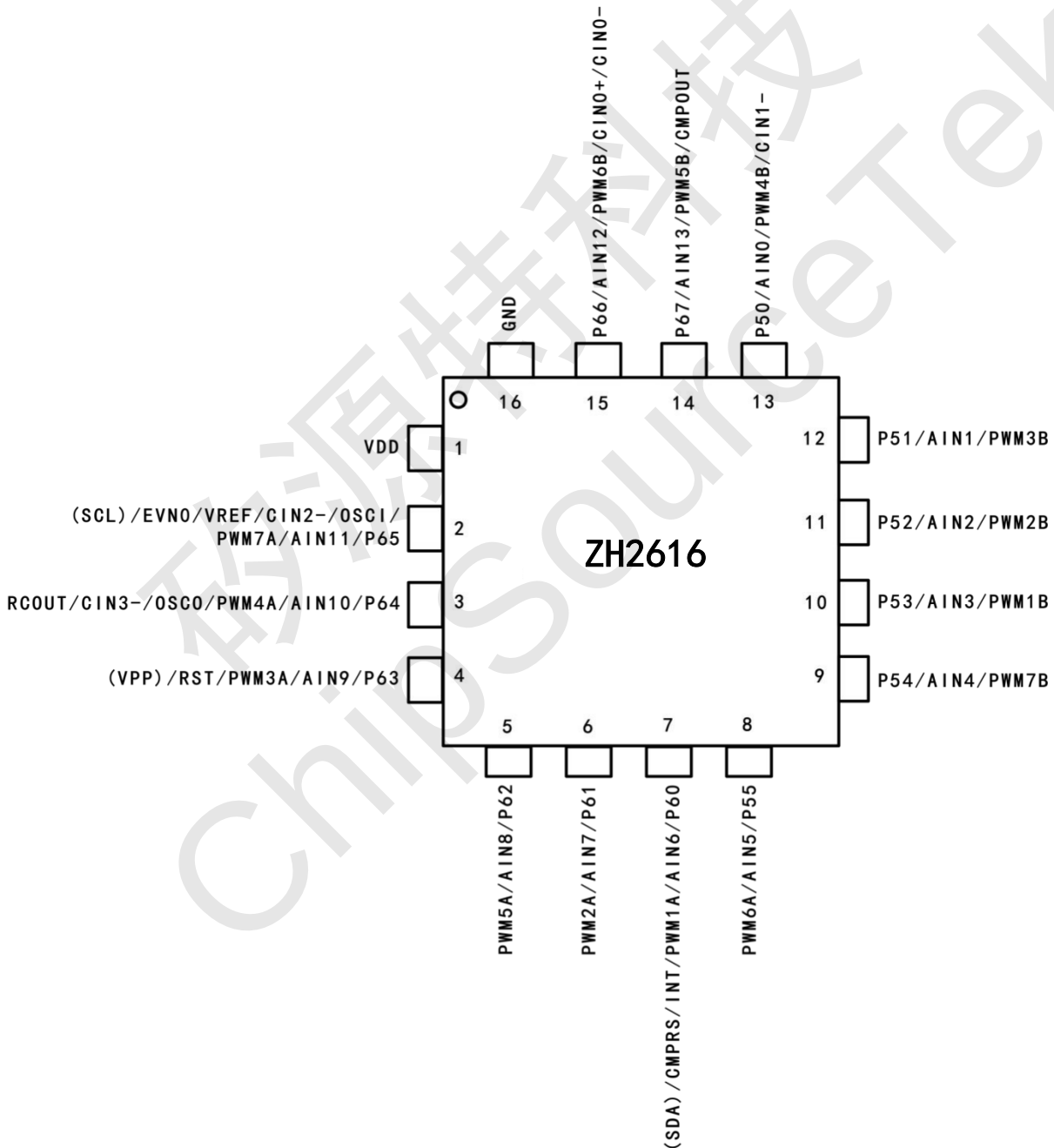
ZH2616-QFN16 脚位图
