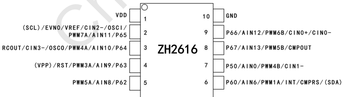
ZH2616-10PIN 脚位图
