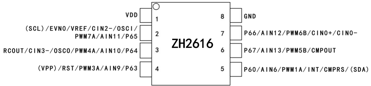
ZH2616-8PIN 脚位图
