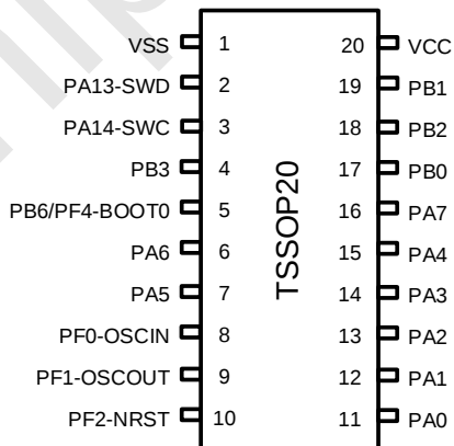
图 3-4 TSSOP20 Pinout1 ZH32F002AF15P
