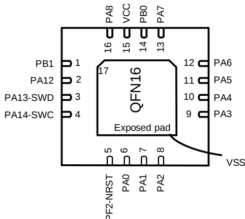
图 3-5 QFN16 Pinout1 ZH32F002AW15U
