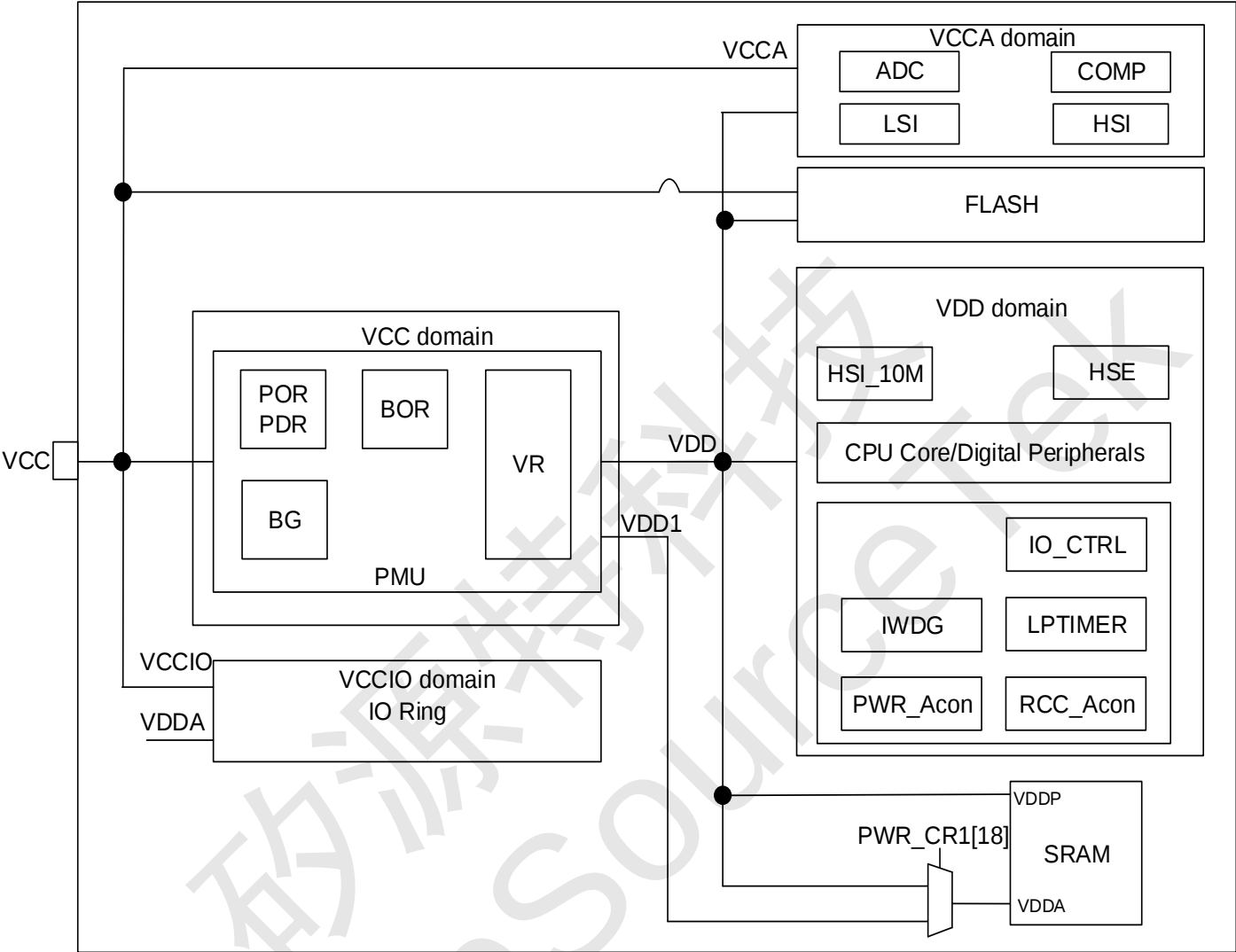
图 2-2 电源框图
