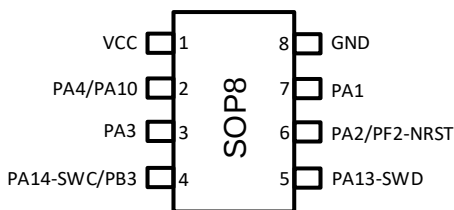
图 3-1 SOP8 Pinout1 ZH32F002AL15S
