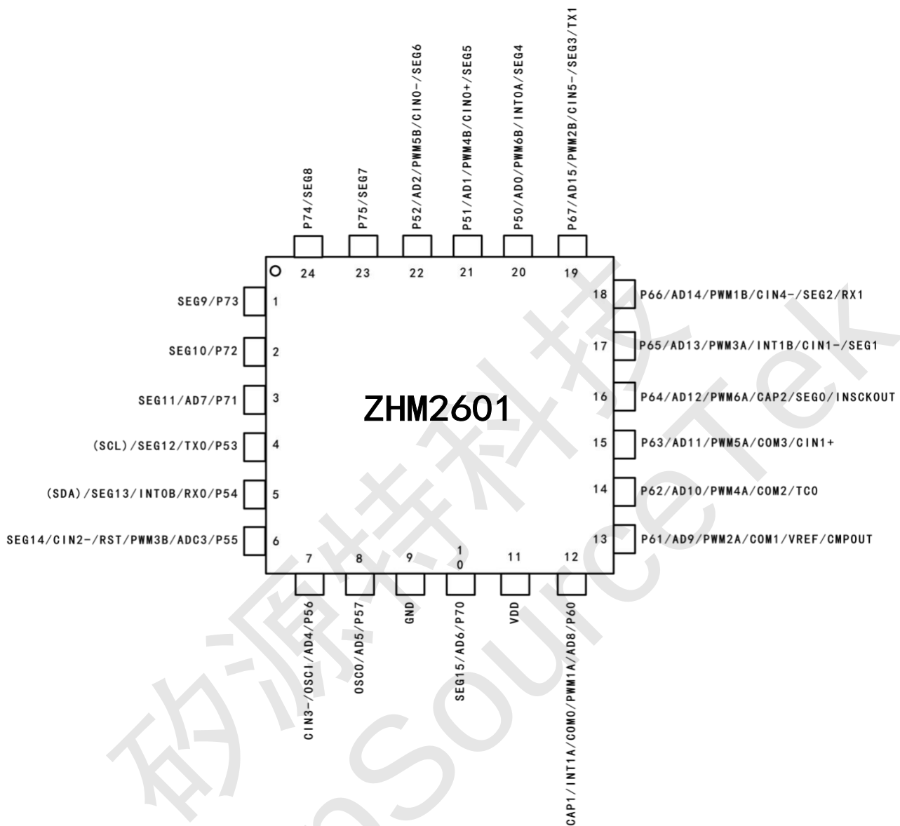
ZHM2601-QFN24 脚位图
