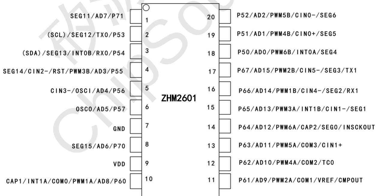
ZHM2601-TSSOP20 脚位图
