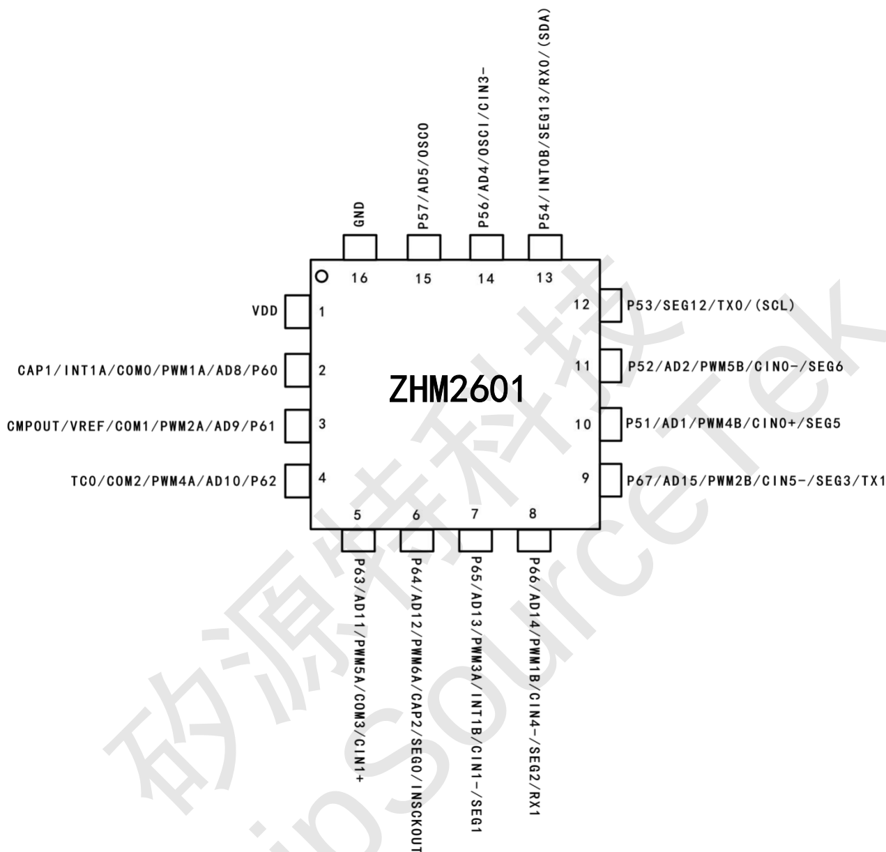
ZHM2601-QFN16 脚位图
