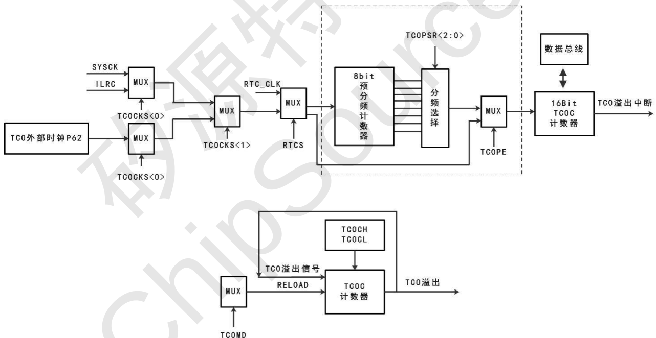
TC0 结构框图
