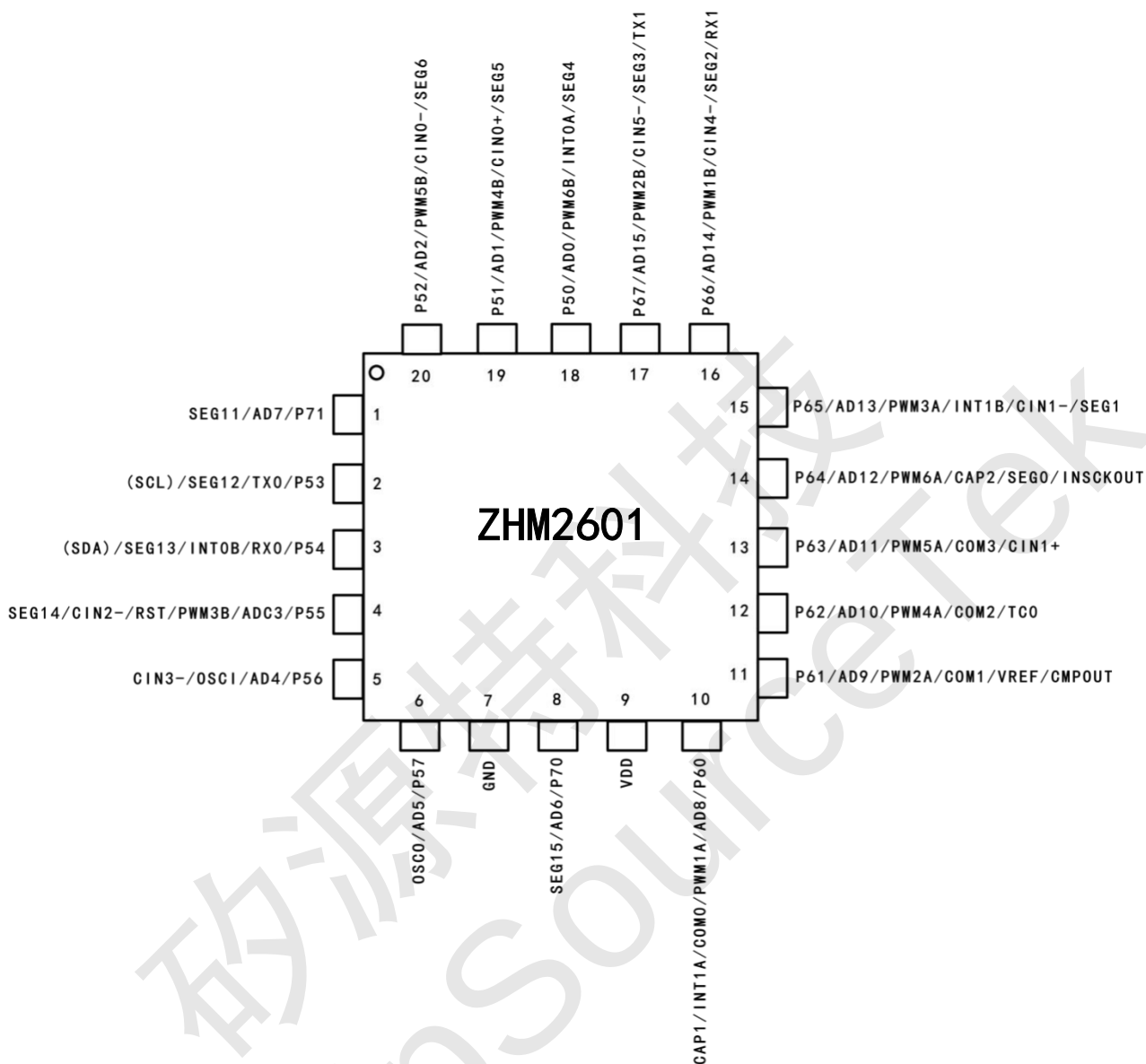
ZHM2601-QFN20 脚位图
