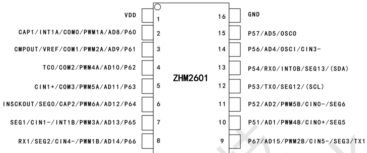
ZHM2601-SOP16 脚位图
