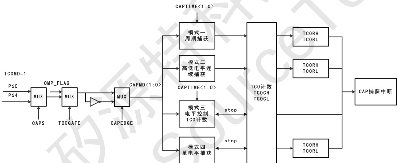
TCO 捕获模式结构框图
