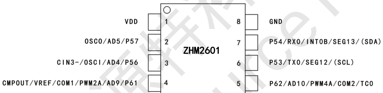
ZHM2601-SOP8 脚位图
