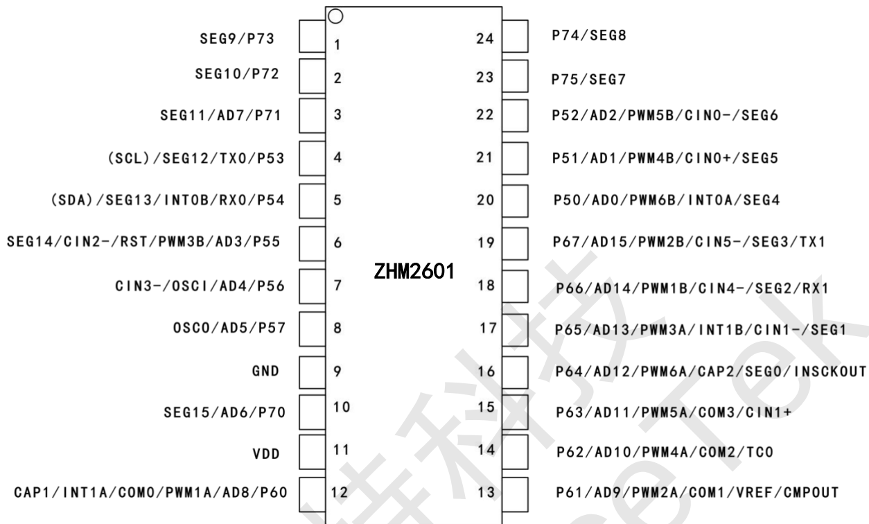
ZHM2601-TSSOP24 脚位图
