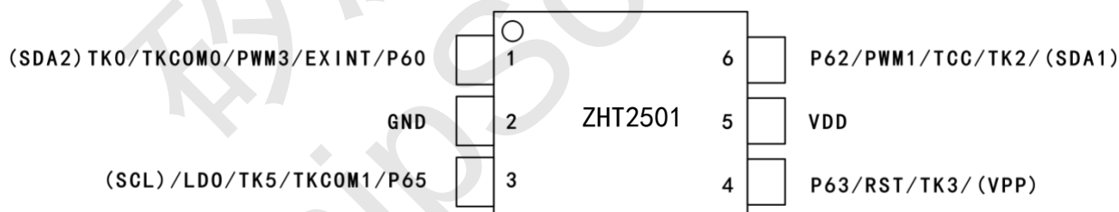
ZHT2501-6PIN 脚位图
