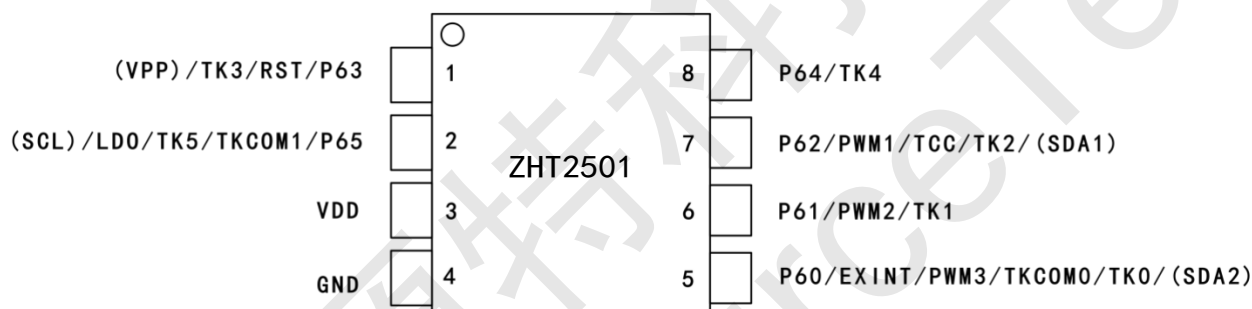
ZHT2501-8PIN 脚位图
