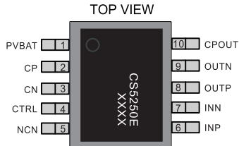
CS5250E(ESOP10 PACKAGE)
