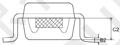
SOT23-3L
