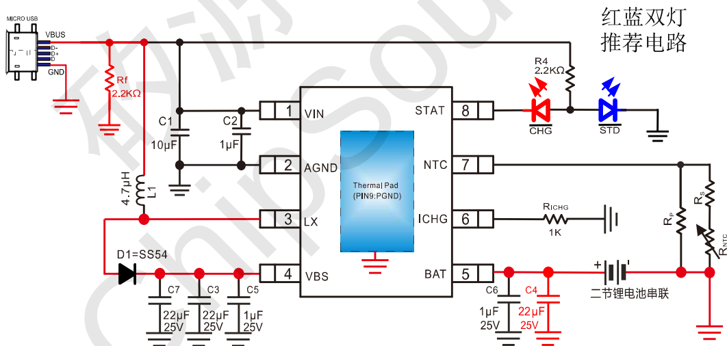
CST5090EA 应用电路图
