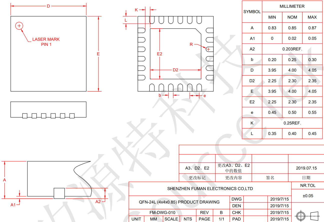
图 2 FM5841 封装尺寸说明 (QFN24_4X4)
