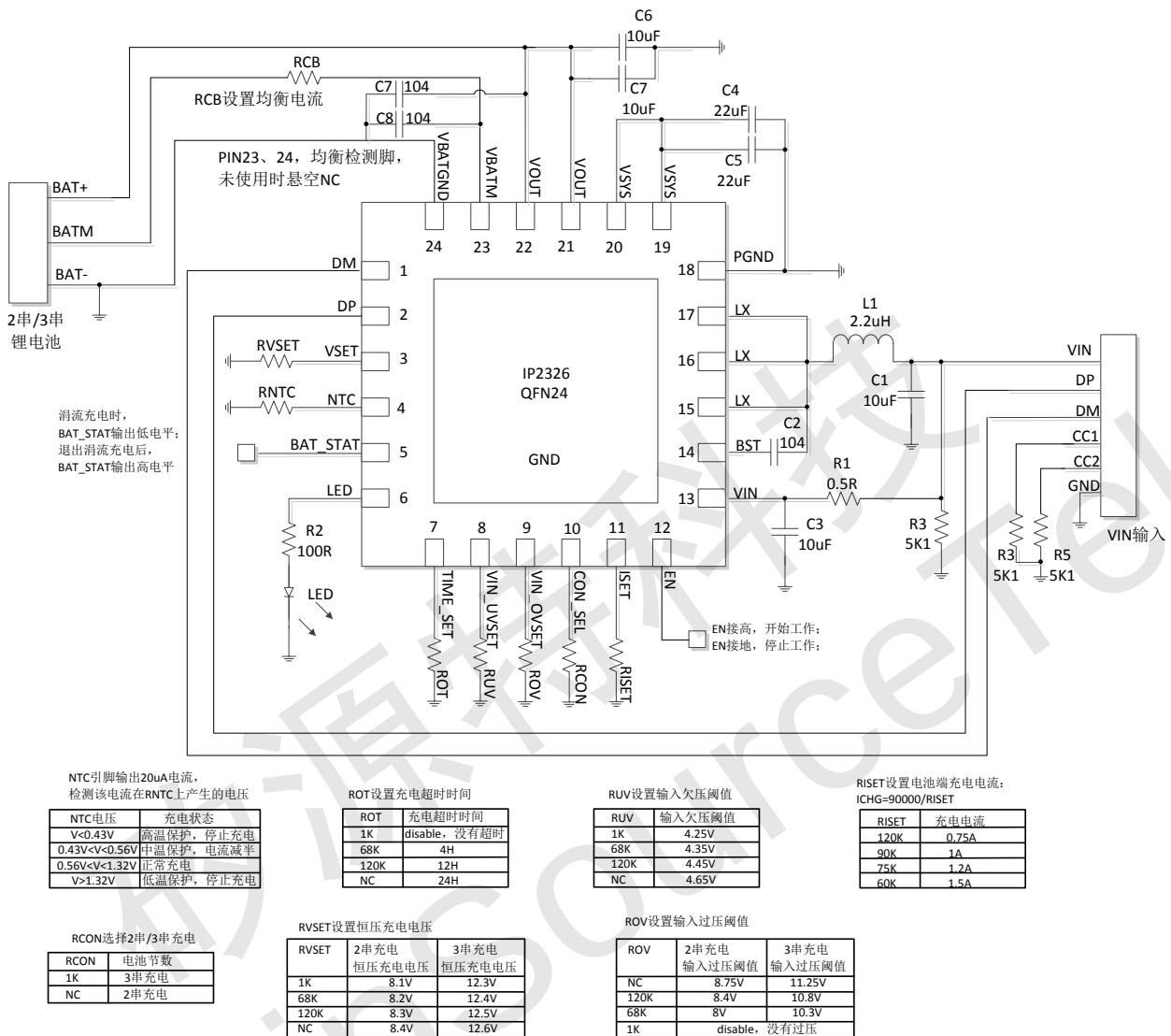
图 5 典型应用原理图
