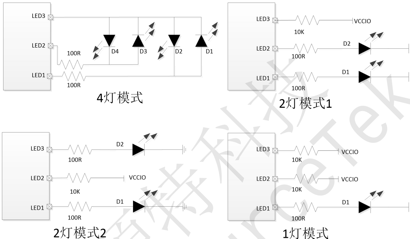
图9 4、2、1 LED 连接方式
