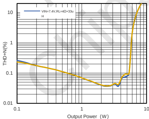
图12. 7.4V电压、4Ω负载输出功率和THD+N
