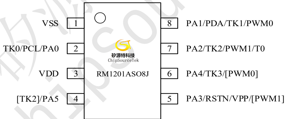
RM1201ASO8J (SOP8)
