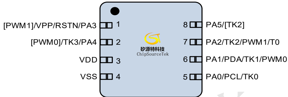
RM1201ADF8A (DFN8)
