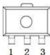
SOT89-3
