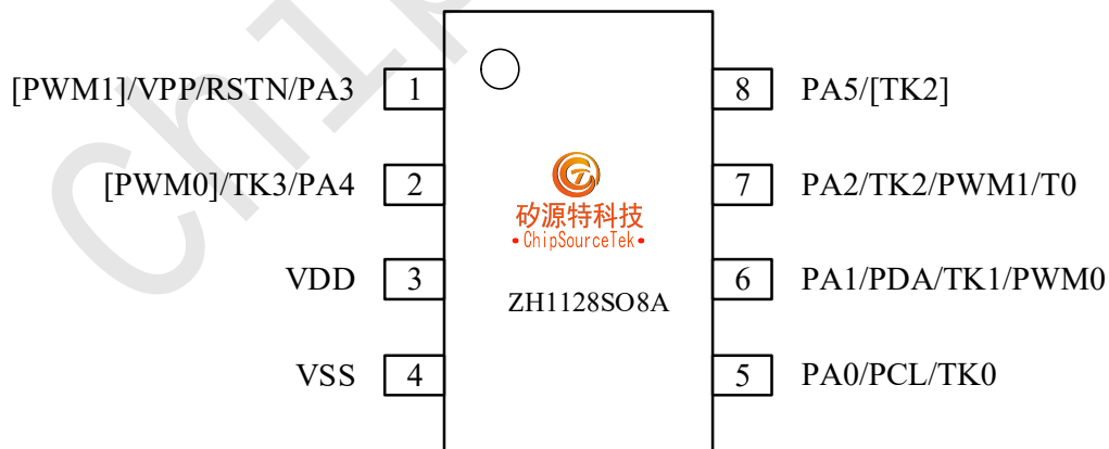
ZH1128SO8A (SOP8)
