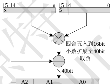
Figure 45 有符号小数乘减带四舍五入
