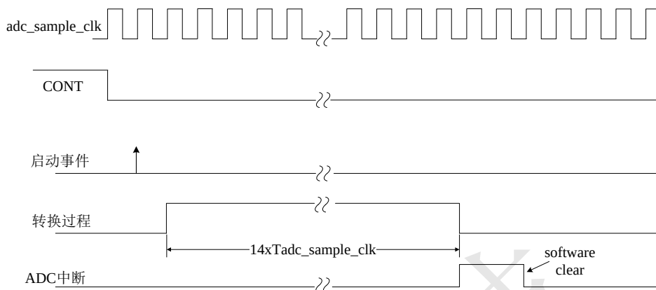
Figure 165 单次 ADC 时序图
