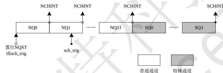
Figure 169 特殊通道序列外部触发方式
