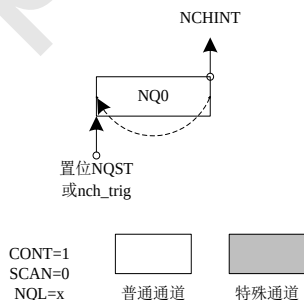
Figure 175 普通通道连续转换+非扫描模式
