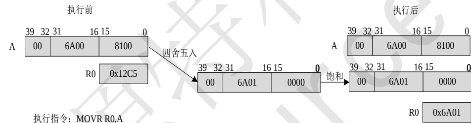
Figure 25 MOVR Rd,A 指令(例 d)
