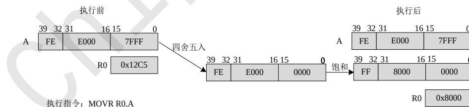
Figure 22 MOVR Rd,A 指令(例 a)
