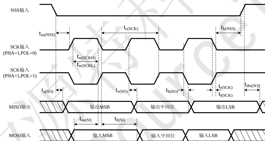
Figure 210 SPI 时序图（从模式，PHA=1）
