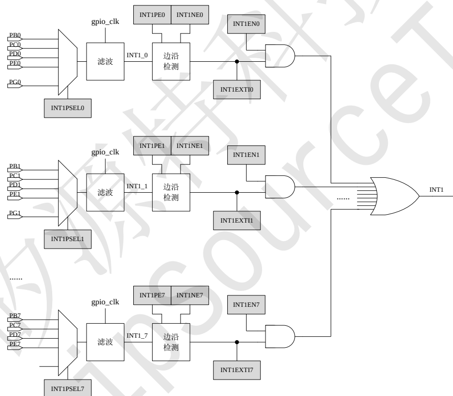
Figure 202 INT1 中断
