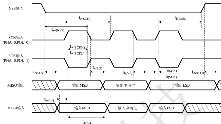
Figure 209 SPI 时序图（从模式，PHA=0）
