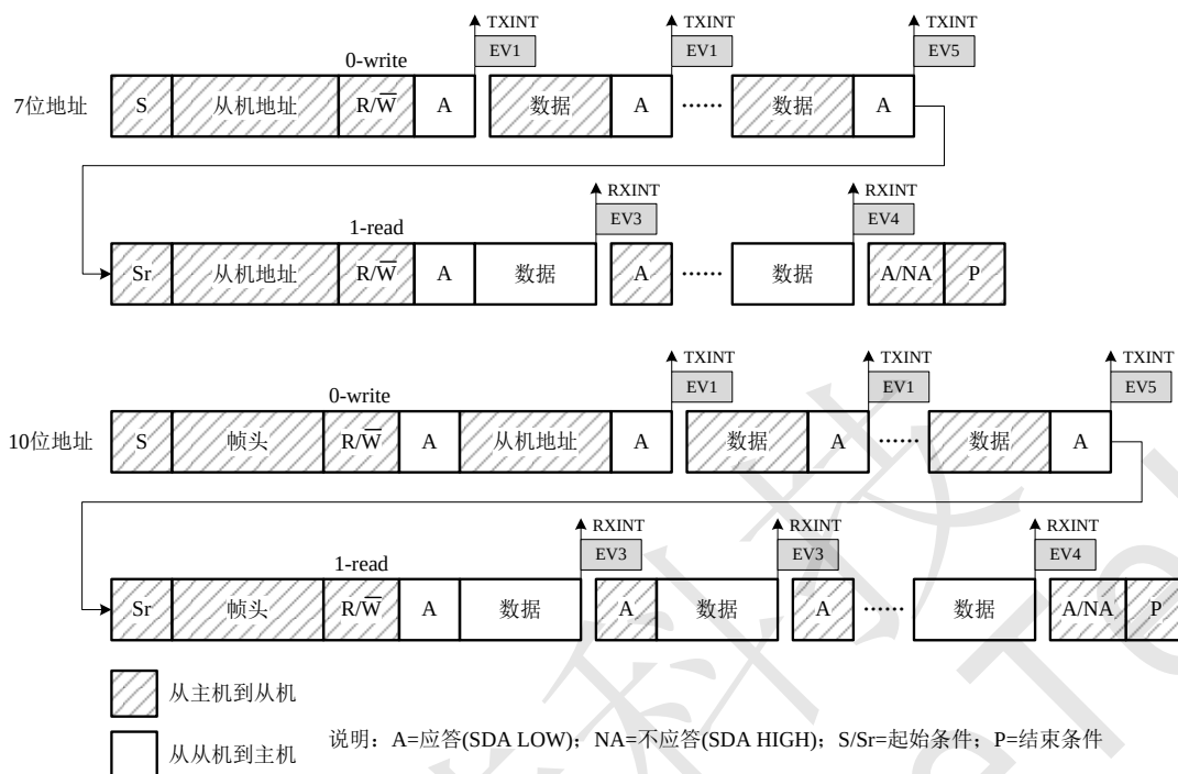
Figure 149 主机混合模式
