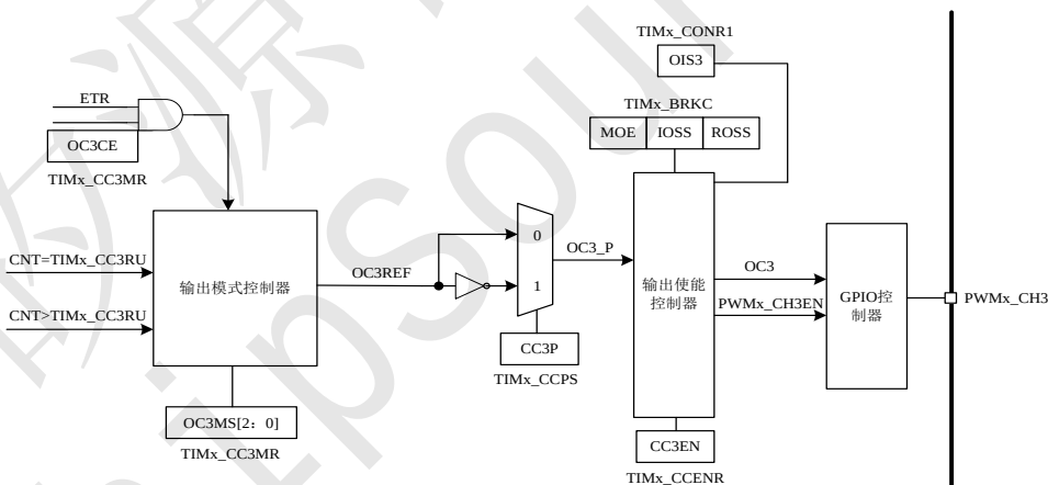
Figure 96 通道 CC3 输出控制
