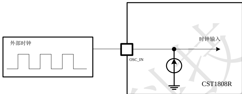
Figure 205 外部时钟输入 OSC_IN 连接示意图
