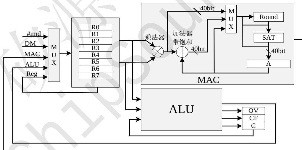
Figure 14 数据运算器框图
