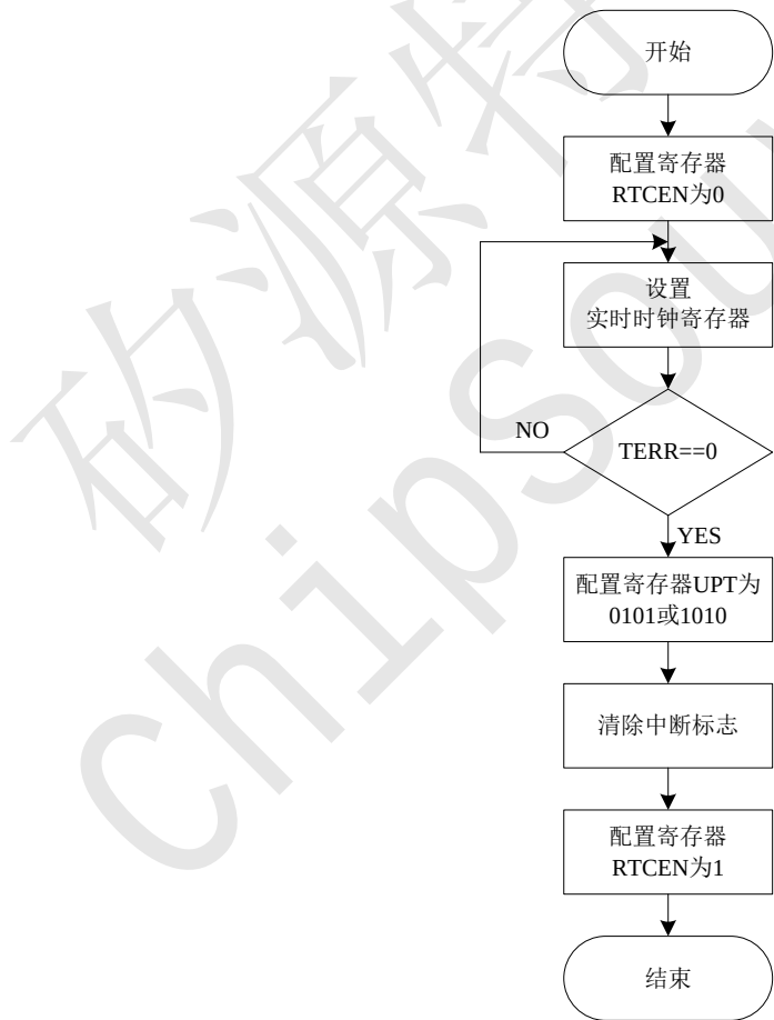
Figure 58 RTC 初始化流程
