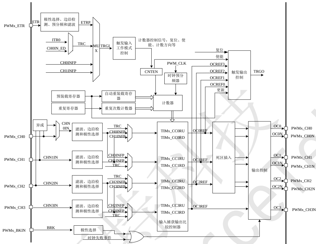
Figure 75 CST1808R 高级定时器 (TIMx/PWMx) 框图
