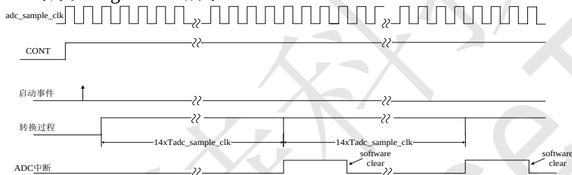
Figure 166 连续 ADC 时序图
