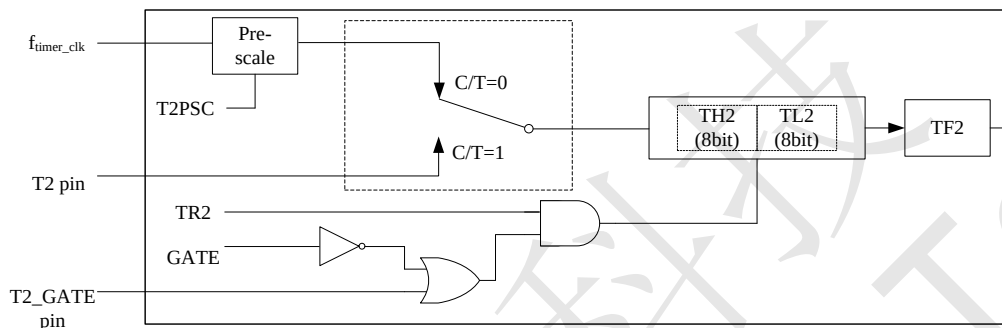
Figure 72 Timer2 模式 1 实现框图
