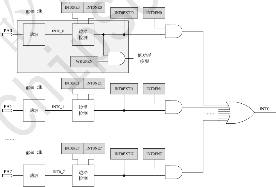
Figure 201 INT0 中断
