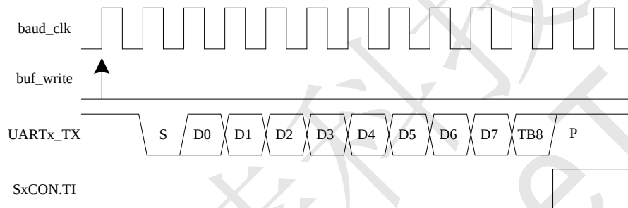
Figure 127 UART 模式 2 发送时序
