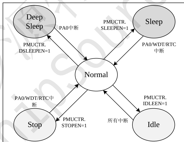
Figure 8 CST1808R 工作模式切换场景图
