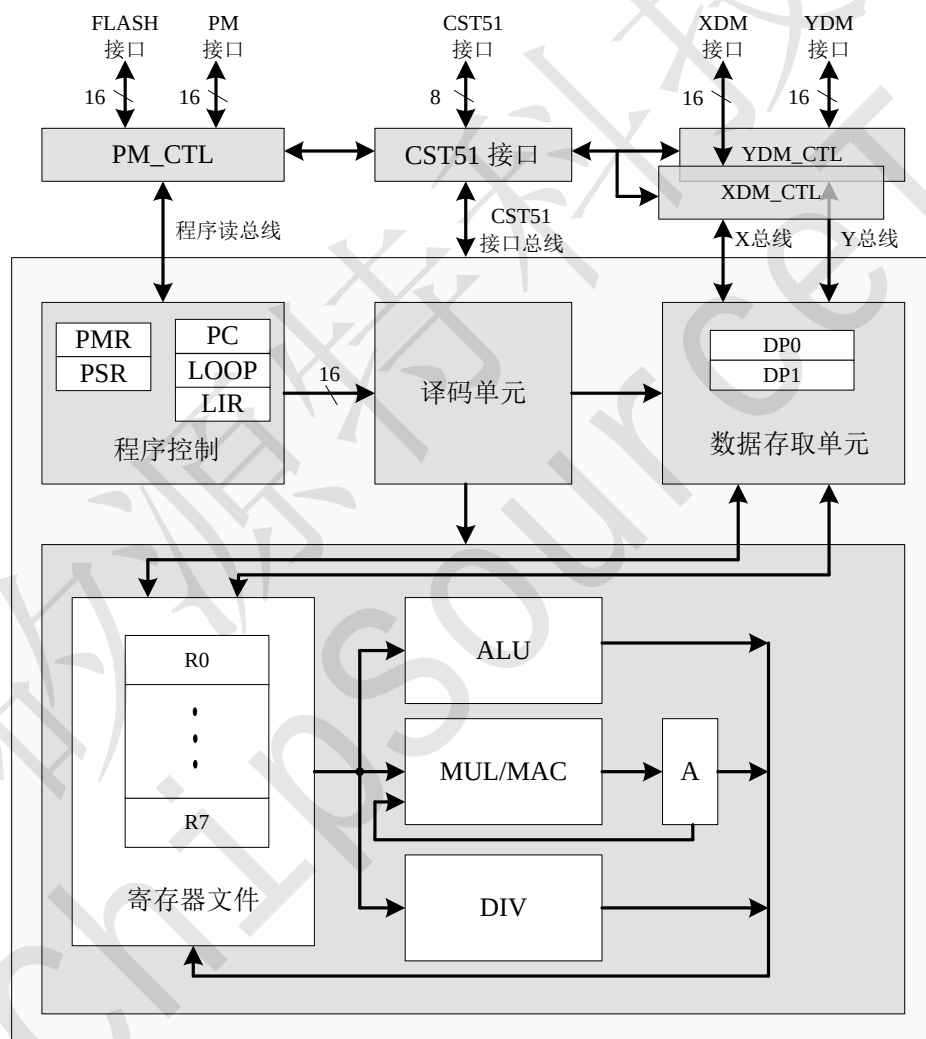
Figure 13 CST018 DSP 核框图
