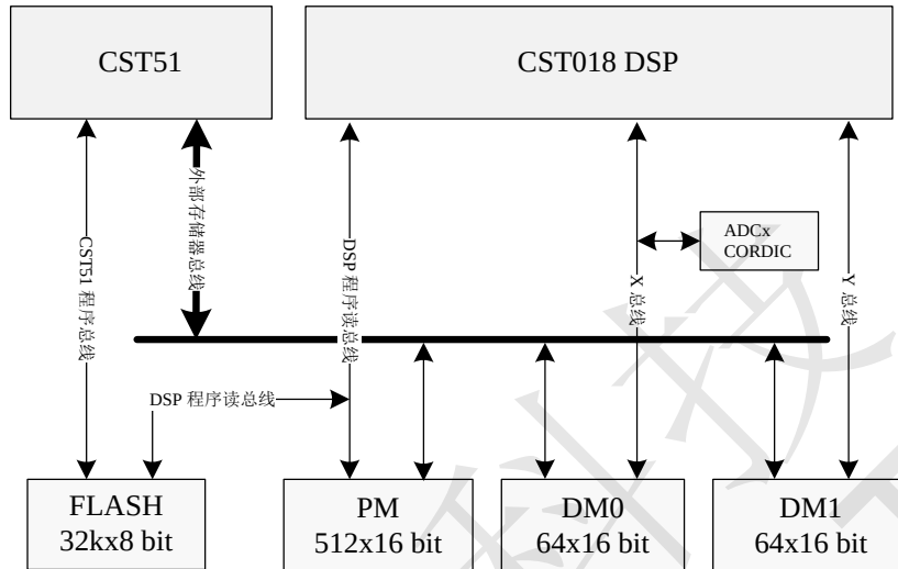
Figure 55 CST018 DSP 存储器分布图
