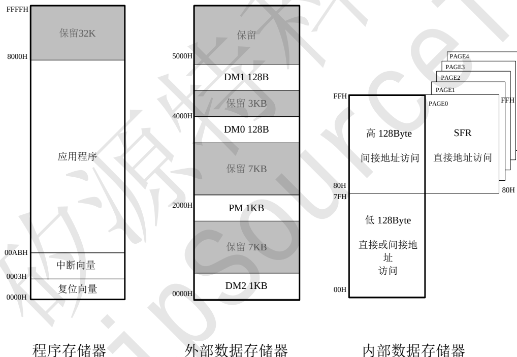
Figure 52 CST51 存储器分布图
