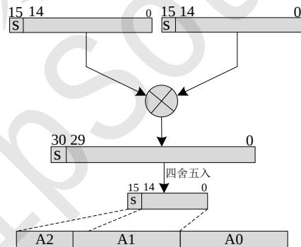
Figure 39 有符号小数相乘带四舍五入
