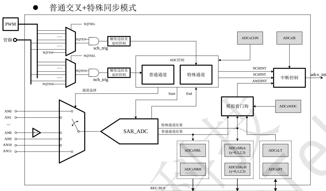
Figure 159 ADC 结构框图
