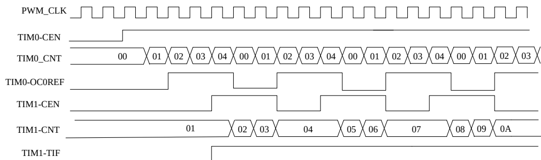
Figure 117 TIM0 的 OC0REF 控制 TIM1 计数器计数
