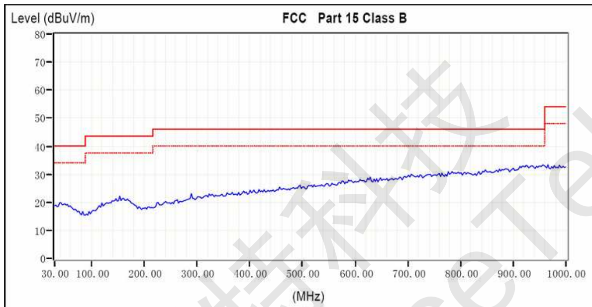
图5 EMI 测试频谱图
