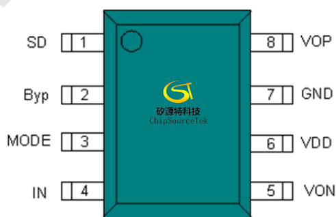
图 2 2018A 管脚定义
