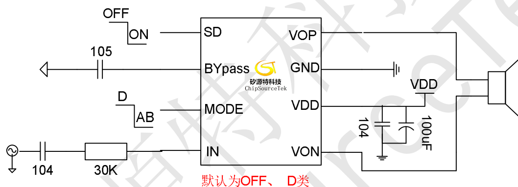
图 1 2018A 典型应用电路
